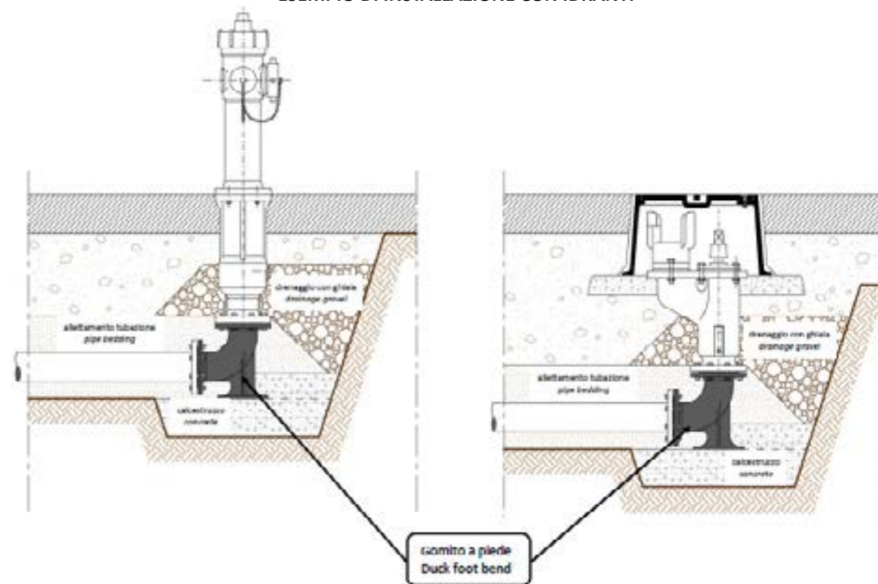
ESEMPIO DI INSTALLAZIONE CON IDRANTI
